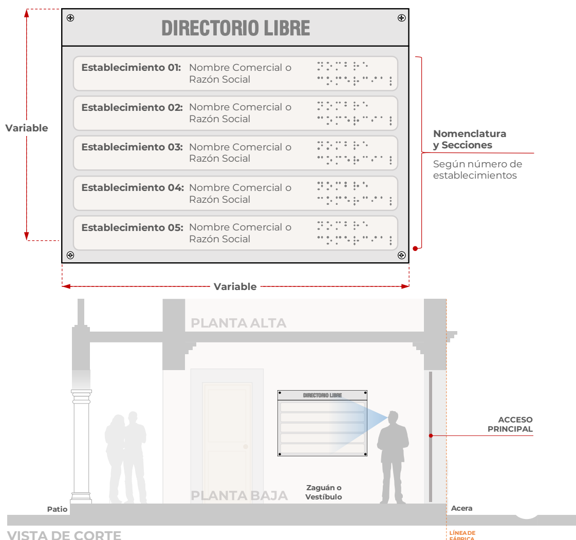
Gráfico 7: Directorio libre en establecimientos con acceso compartido.
