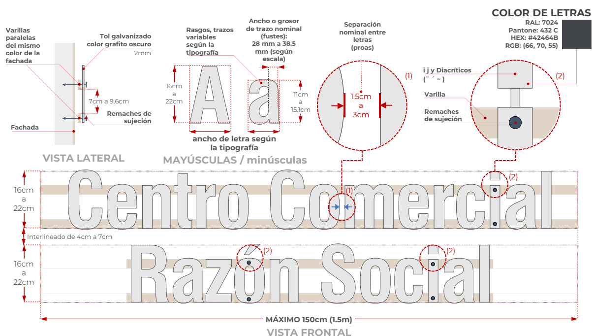
Gráfico 8: Rotulación para centros y pasajes comerciales.
