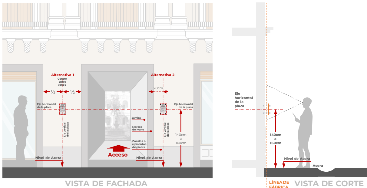
Gráfico 11: Implantación de Directorio Único QR.
