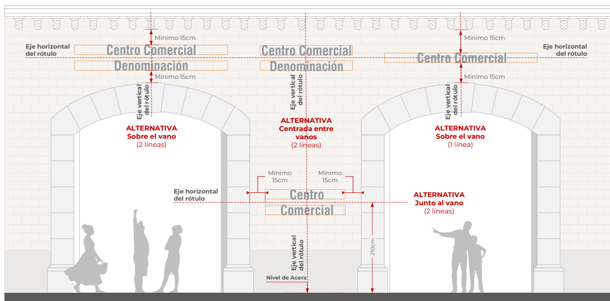
Gráfico 9: Implantación de Rótulo Tipográfico para Centros y Pasajes Comerciales.
