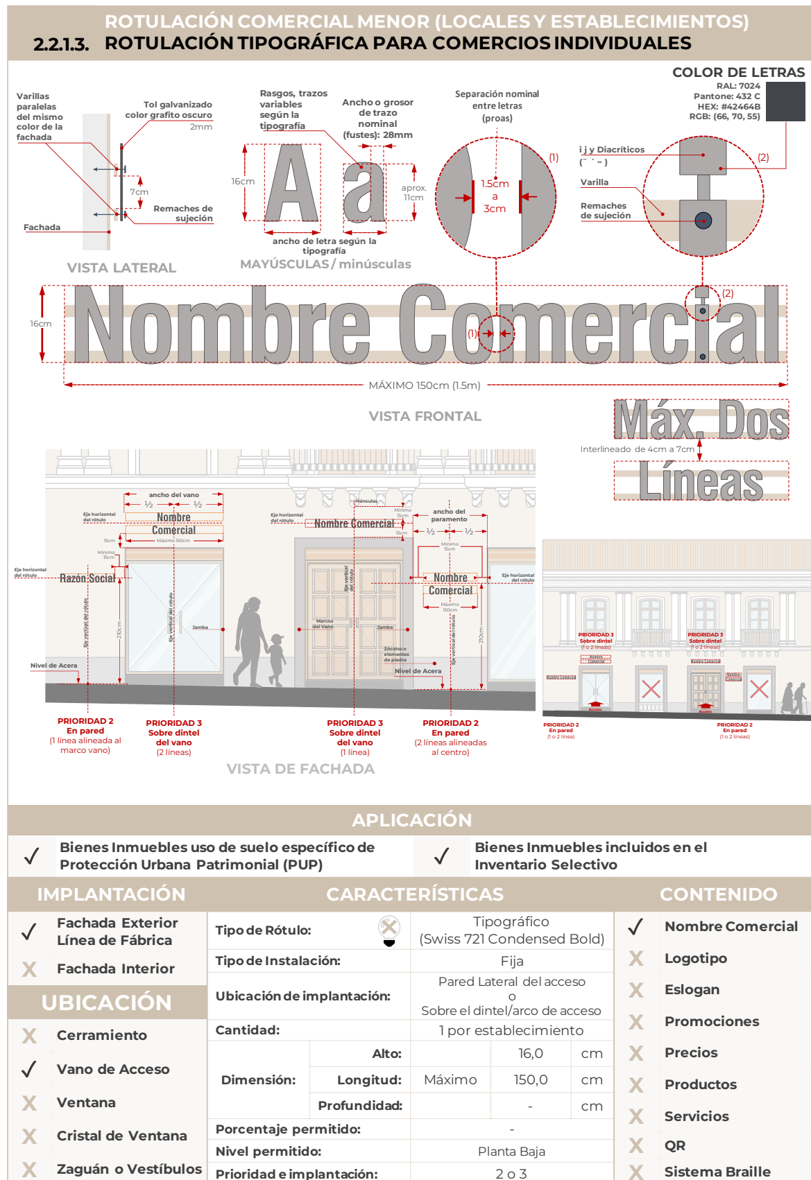
Ficha Técnica 13: Rotulación tipográfica para comercios individuales.
