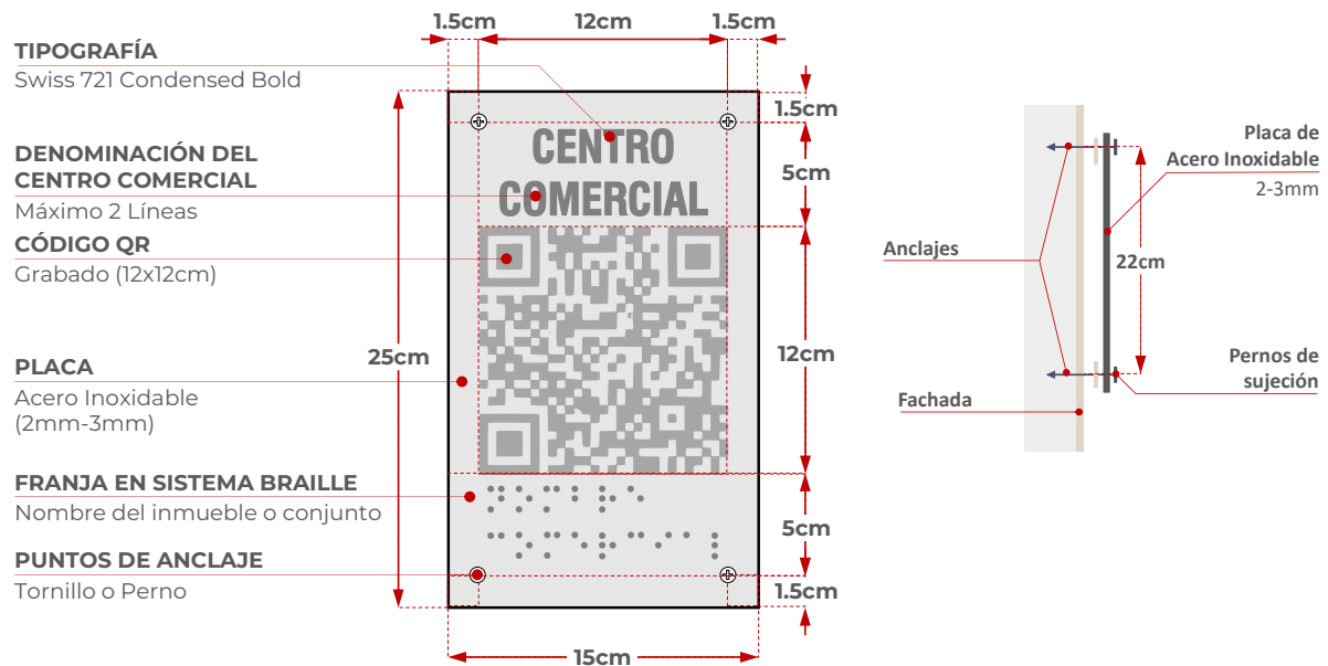
Gráfico 10: Directorio único para centros comerciales.
