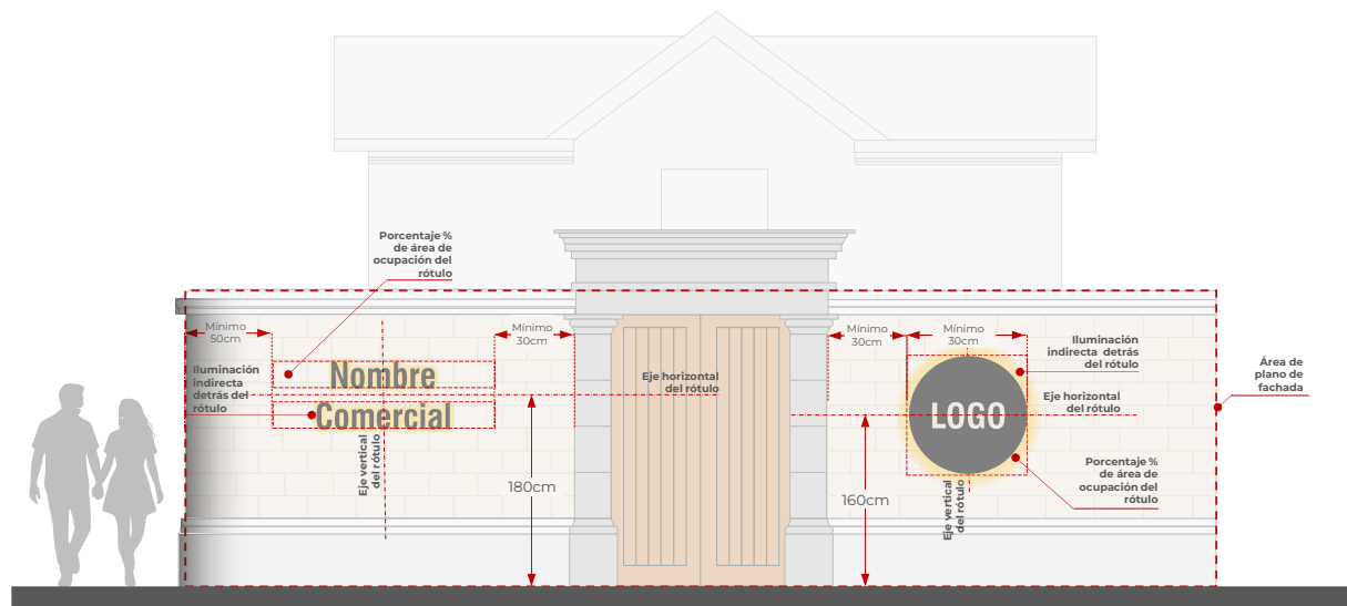
Gráfico 3: Rotulación de identificación comercial en bienes inmuebles incluidos en el inventario selectivo.
